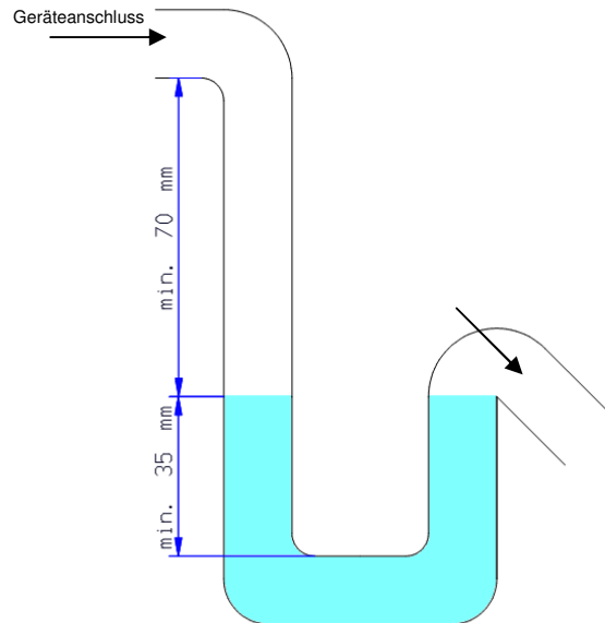
Abbildung: Mindestmaße Siphon
