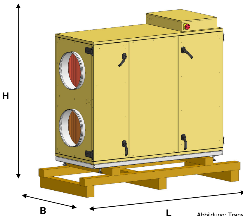
Abbildung: Transportmaße Suprabox
