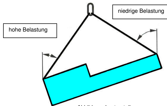
Abbildung: Lastverteilung
