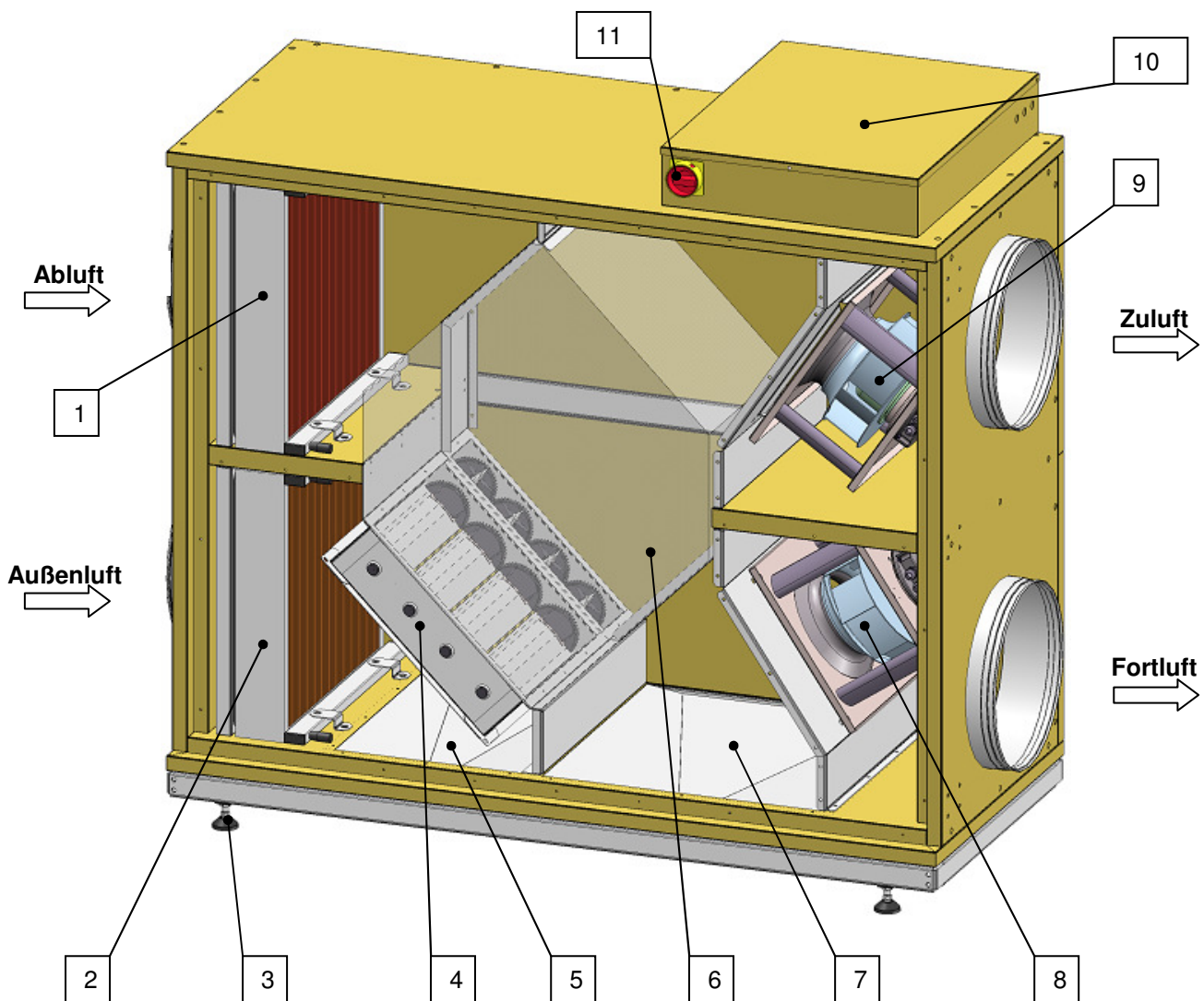
Abbildung: Geräteübersichtszeichnung
