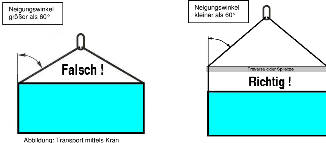
Abbildung: Transport mittels Kran
